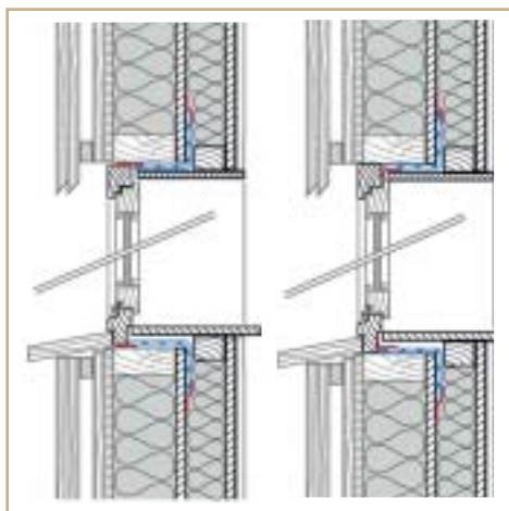
Napojení na boku okenního rámu pomocí TESCO PROFILU
