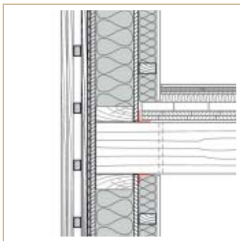
Napojení trámu, který prochází neprodyšnou izolační vrstvou, pomocí TESCO PROFILU
