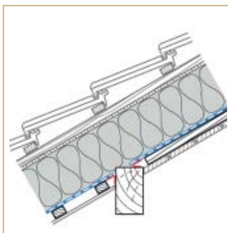
Na hoblovanou střední vaznici napojuje pomocí TESCON PROFILU
