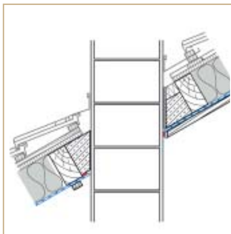
Napojení na omítnutý komín pomocí ORCON F nebo ECO COLL.
